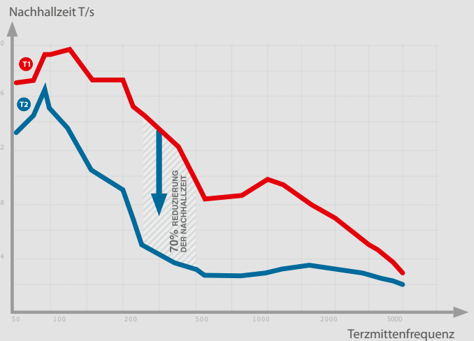
T1 Mittelwert der Nachhallzeit ohne Absorber T2 Mittelwert der Nachhallzeit mit xilent-Akustik-Panel
